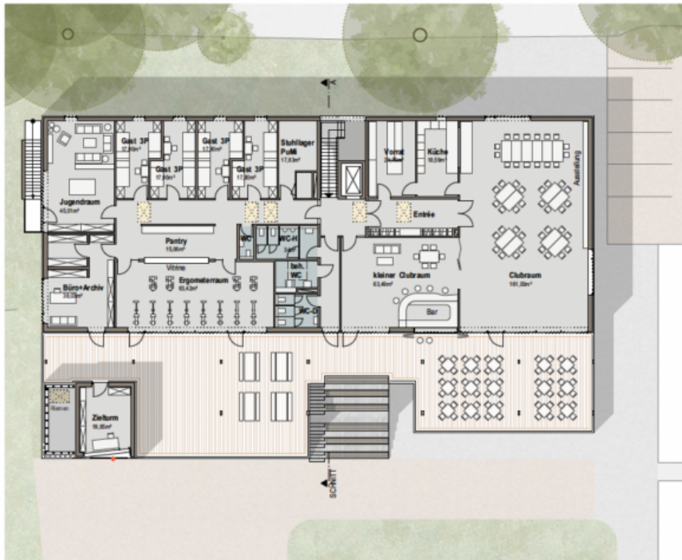
OBERGESCHOSS M. 1:300
